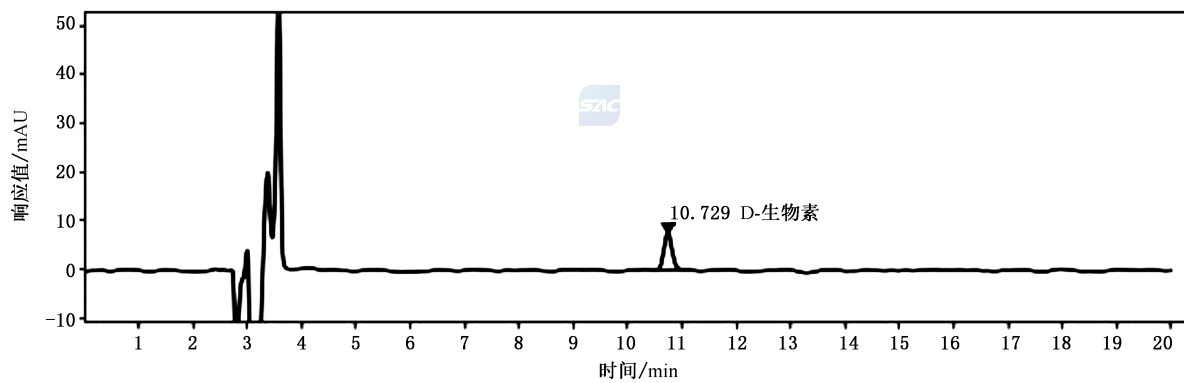
图 A.1 D-生物素标准溶液(10 \mu\text{g}/\text{mL} )的液相色谱图
